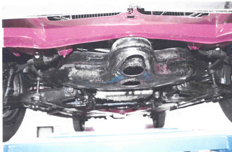
Bild 8 Aggregate original und überholt
